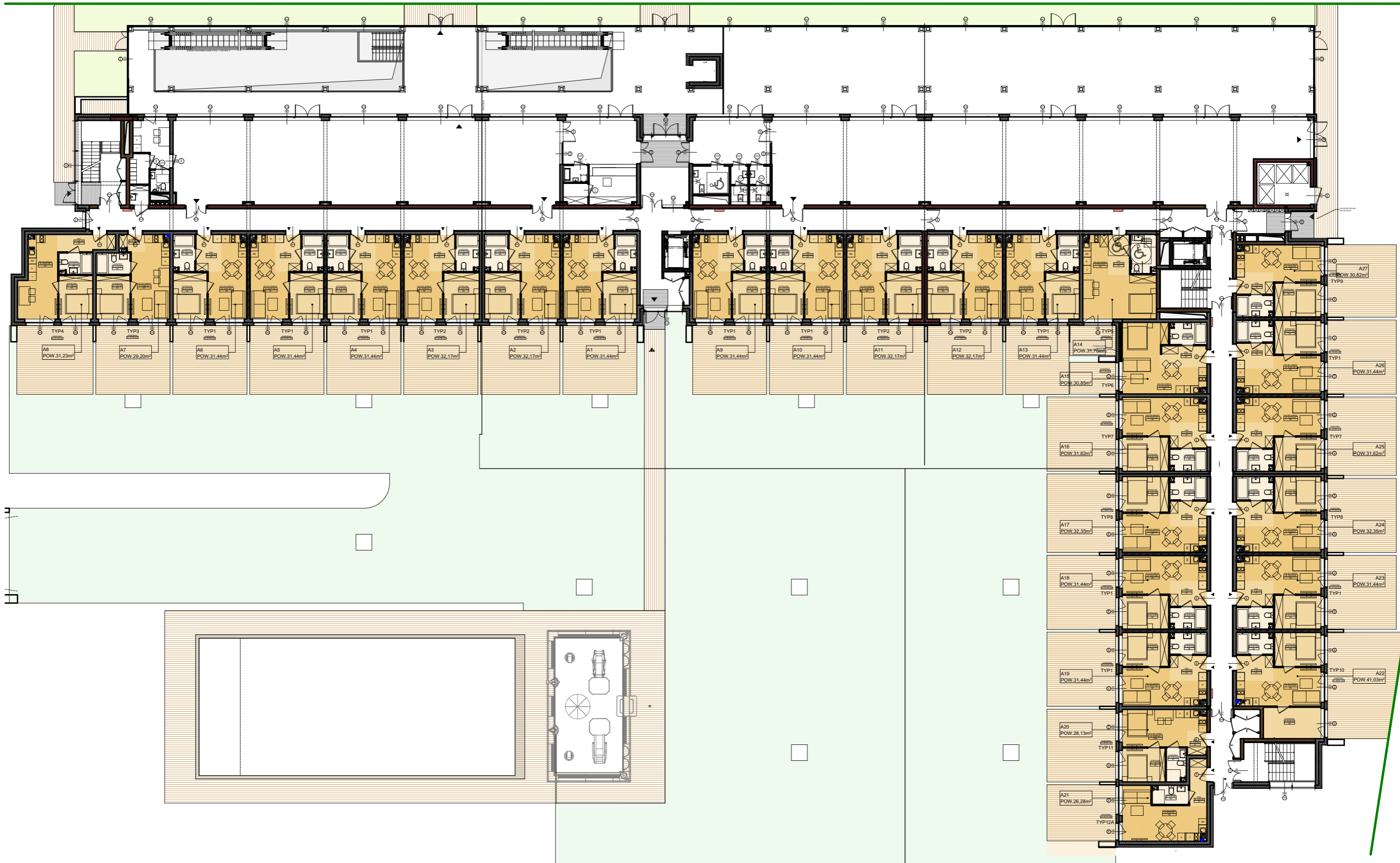
RZUT PARTERU
